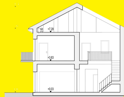
SEZIONE
