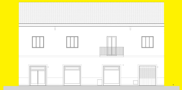
PROSPETTO SUD
